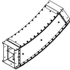
1 m Verlängerung mit 30° Bogen. Wird auch mit 15° (0,50 m) und 45° (1,50 m) geliefert
