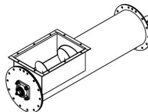
Schneckenfuss, Einlauf/Auslauf SS254
