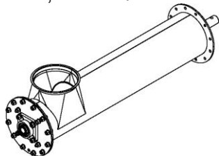
Schneckenfuss, Einlauf/Auslauf SS205
